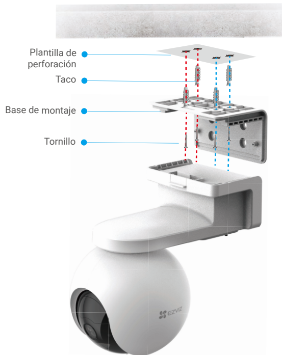
Figura 1. Montaje en techo
